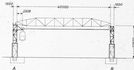
Bild 2. Krananlage, Querschnitt 1:800
