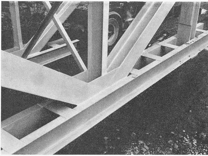
Bild 5. Untergurtnoten
