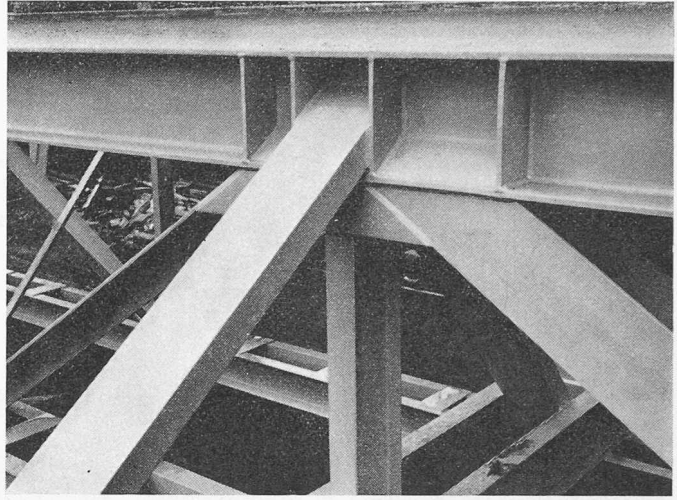
Bild 6. Obergurtnoten
