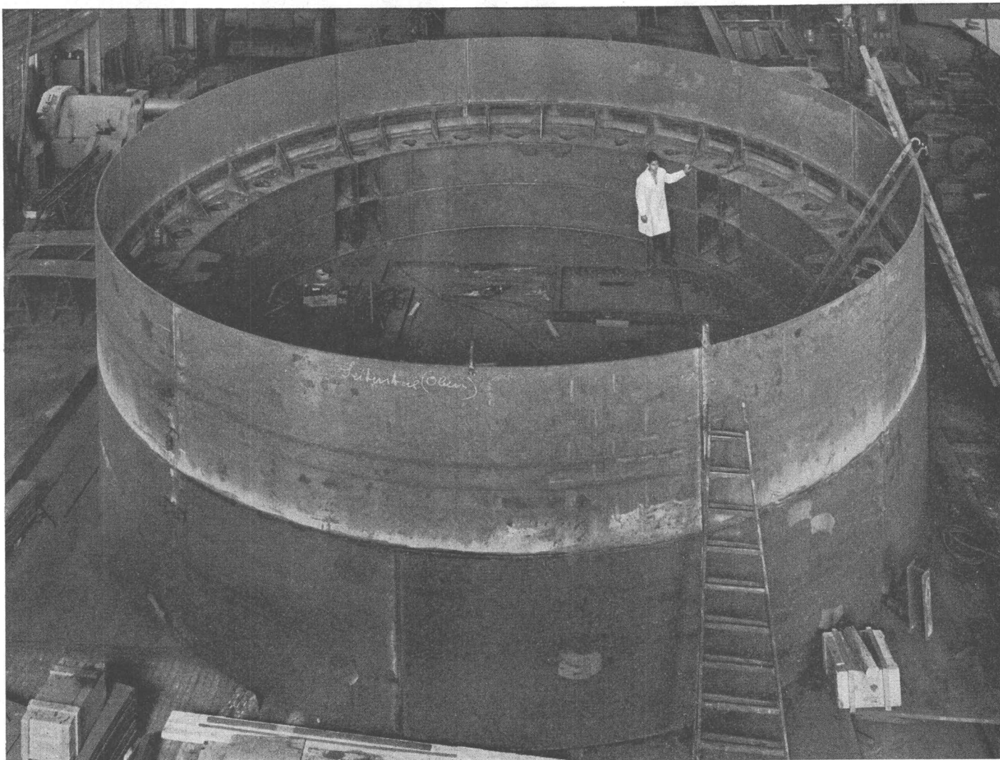
Zusammenbau des hinteren Schildschusses (Schildschwanz) in unseren Werkstätten in Basel
