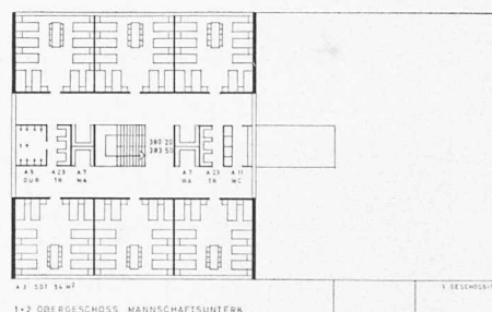
1+2 OBERGESCHOSS MANNSCHAFTSUNTERK
