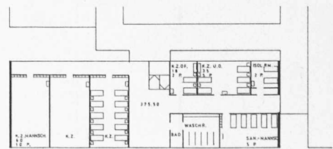
KRANKENABTEILUNG D
