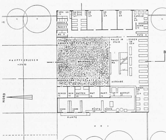
KOMPAGNIE EINHEIT
