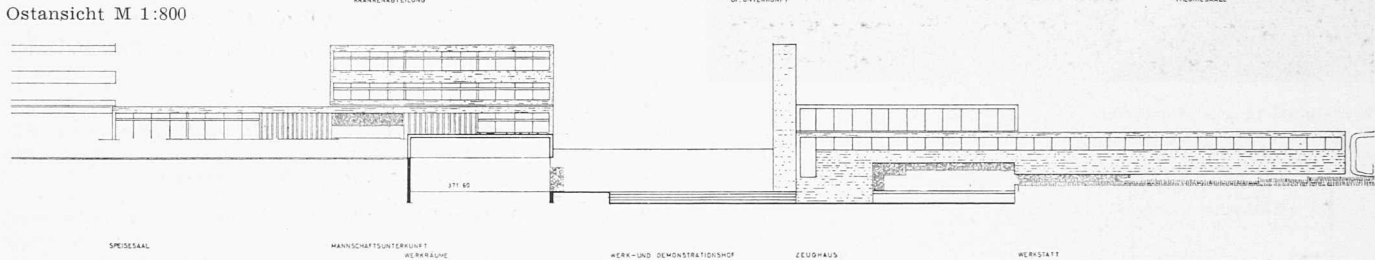
Ostansicht mit Schnitt durch Werkhof M 1:800
