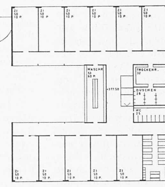
Mannschaftsgebäude Masstab 1:800, links Erdgeschoss, oben Obergeschoss
