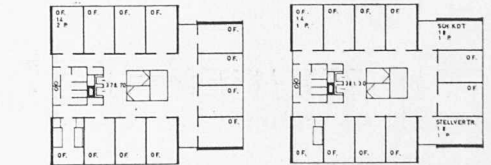
Offiziersunterkunft im ersten und zweiten Obergeschoss
