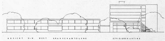
ANSICHT N-W WEST KRANKENABTEILUNG
