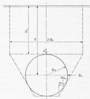
Bild 30. Erddruck nach Terzaghi
