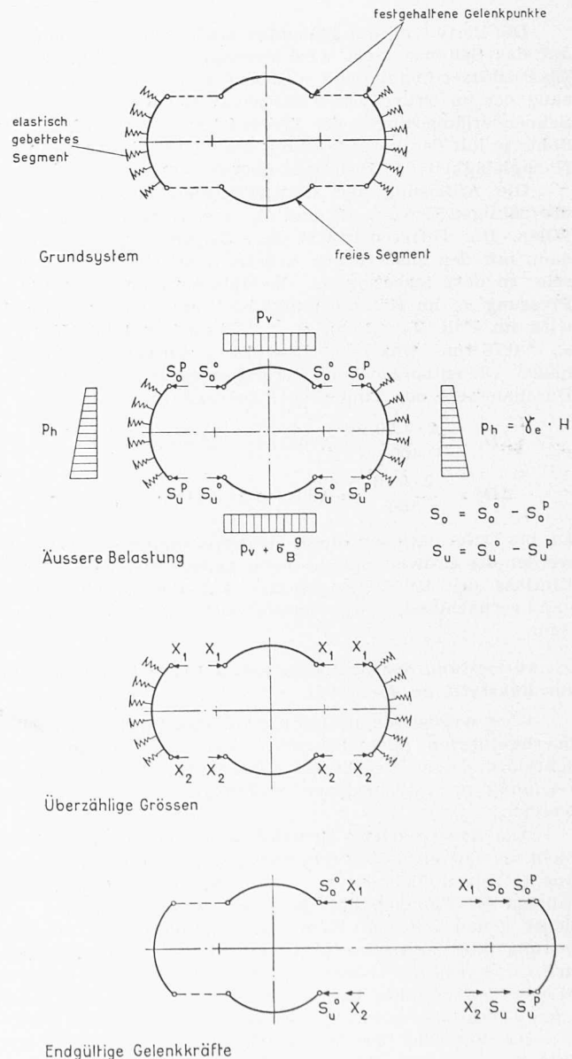
Bild 31. Berechnung des elastisch gebetteten Viergelenkbogens
