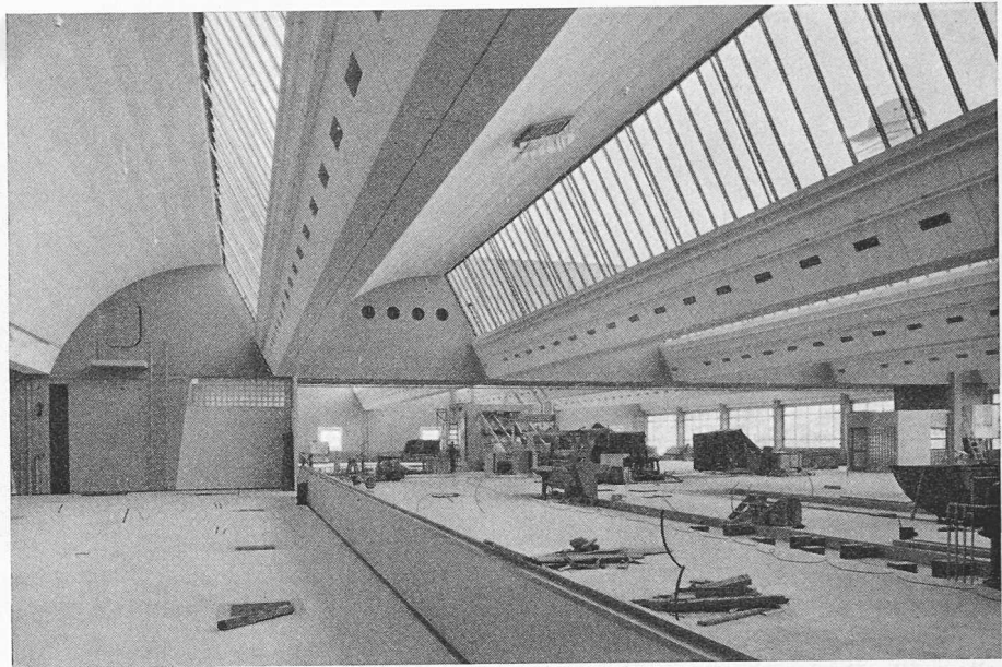
Bilder 12 und 13. Textilfabrik Schild AG in Bern. Grundrissfläche von rund 5000 m 2 , nur eine Stütze in Hallenmitte, vorgespannte Shedschalen von rund 36 m Spannweite, welche auf einem Kastenträger ruhen
