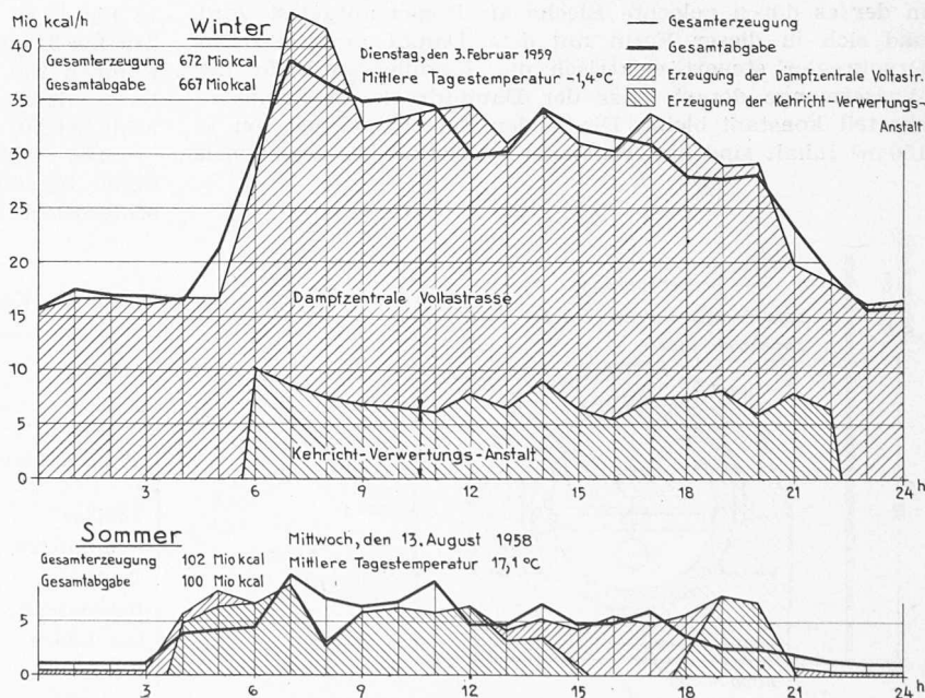
Bild 5. Verlauf der Wärmeenergieerzeugung und des Wärmebezuges während eines Wintertages (3. Februar 1959, mittlere Temperatur -1,4°C) und während eines Sommertages (13. August 1958, mittlere Temperatur 17,5°C)
