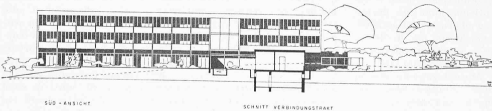
SCHNITT VERBINDUNGSTRAKT
