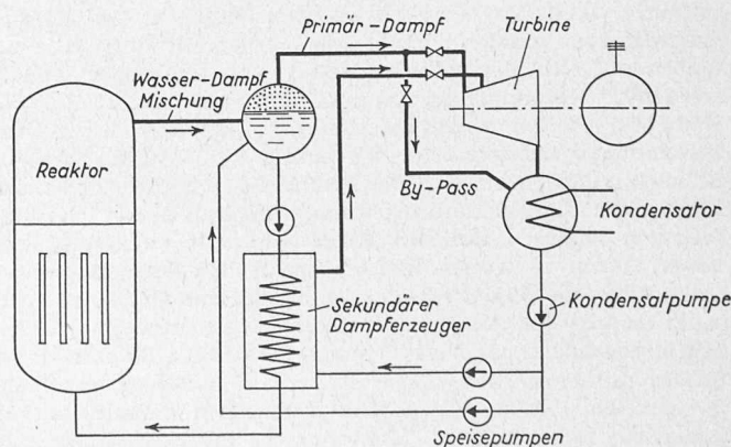
Bild 9 (rechts). Vereinfachtes Schema des Siedewasser-Reaktors mit Doppelkreislauf
