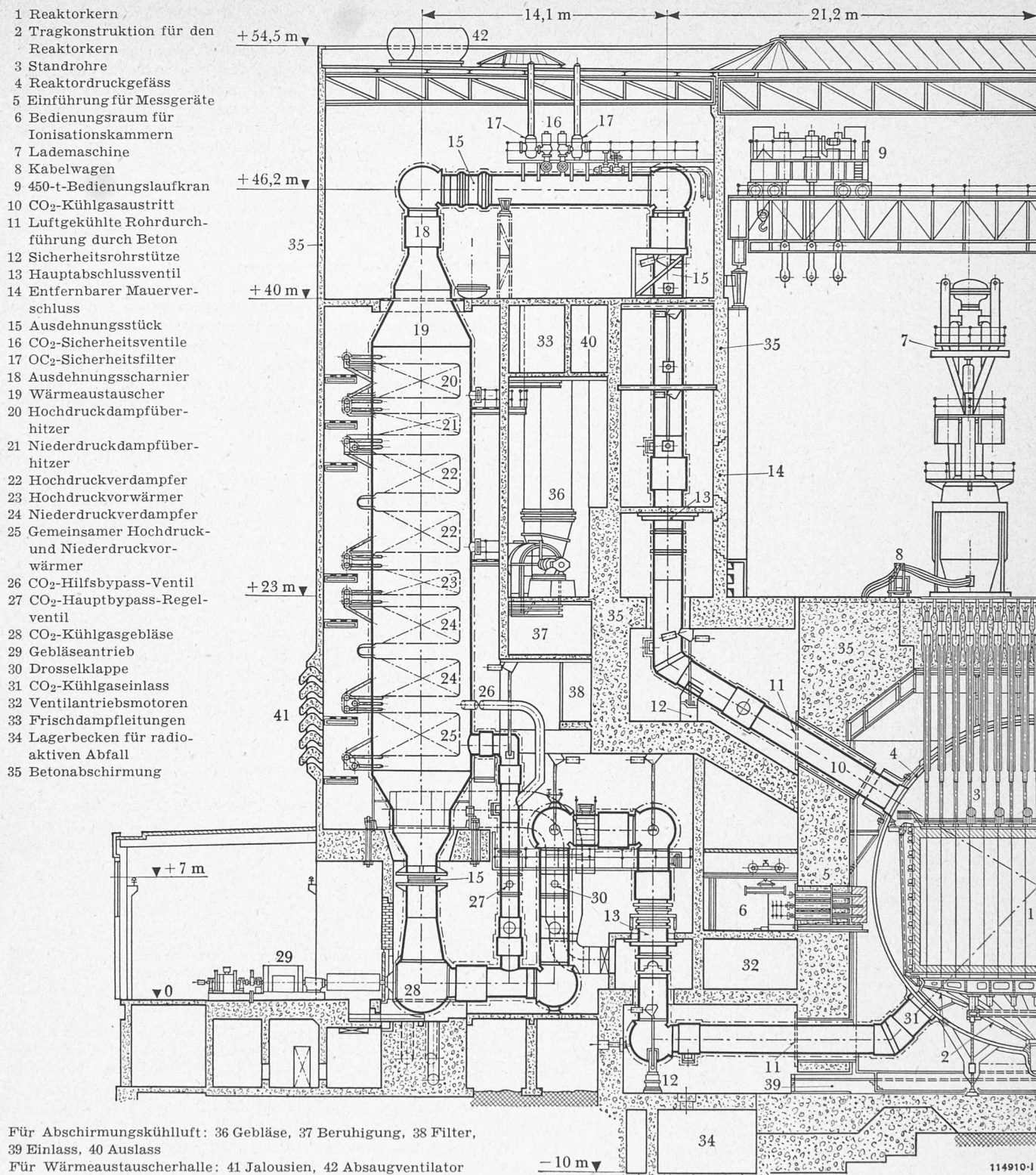
Bild 12. Kernenergie-Kraftwerk Trawsfynydd, Schnitt durch das Reaktorgebäude mit einem der sechs Kühlgas-Kreisläufe. Im Maschensaal dieses Kraftwerkes sind 4 Turbogruppen von je 145 MW Klemmenleistung, Bauart Brown Boveri (Lizenznehmer Richardsons Westgarth & Co. Ltd.), aufgestellt. (Aus «Brown Boveri Mitteilungen», Jan./Febr. 1960, S. 97)
