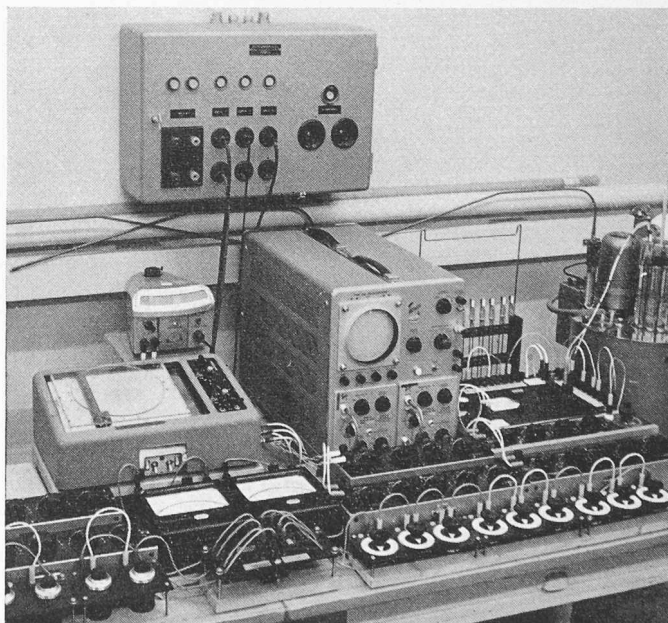
Bild 3. Apparat zur Messung der Wärmeleitfähigkeit von Flüssigkeiten. (Die von dipl. Ing. W. Straumann im Institut für kalorische Apparate und Kältetechnik entwickelte Apparatur gestattet in etwa einer Minute die Wärmeleitfähigkeit einer Flüssigkeit mit einer Genauigkeit von \pm 1\% zu messen.)
