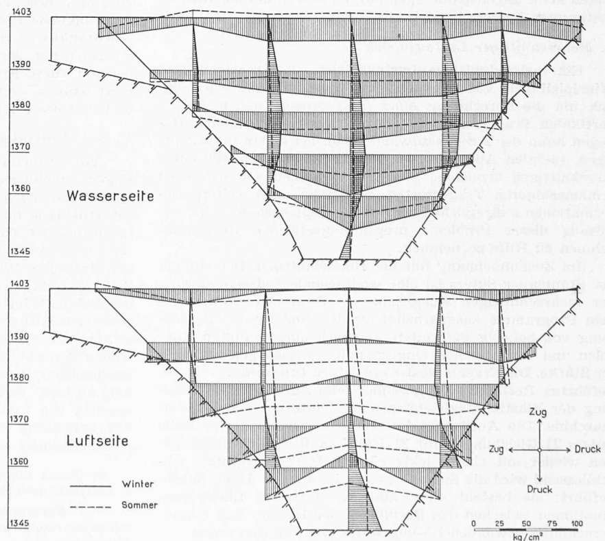
Bild 7. Wasser- und luftseitige Normalspannungen an der Staumauer Sufers auf Grund eines fünfschnittigen radialen Lastausgleichs und für zwei Temperaturzustände bei Vollstau
