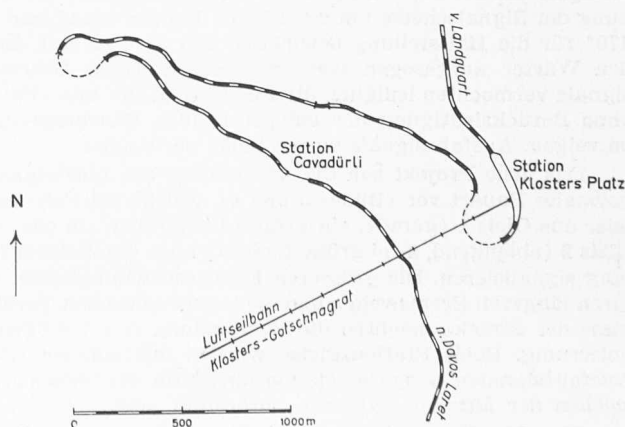
Bild 1. Lageplan 1:3500 der Strecke Klosters-Cavadürli-Laret der Rhätischen Bahn
