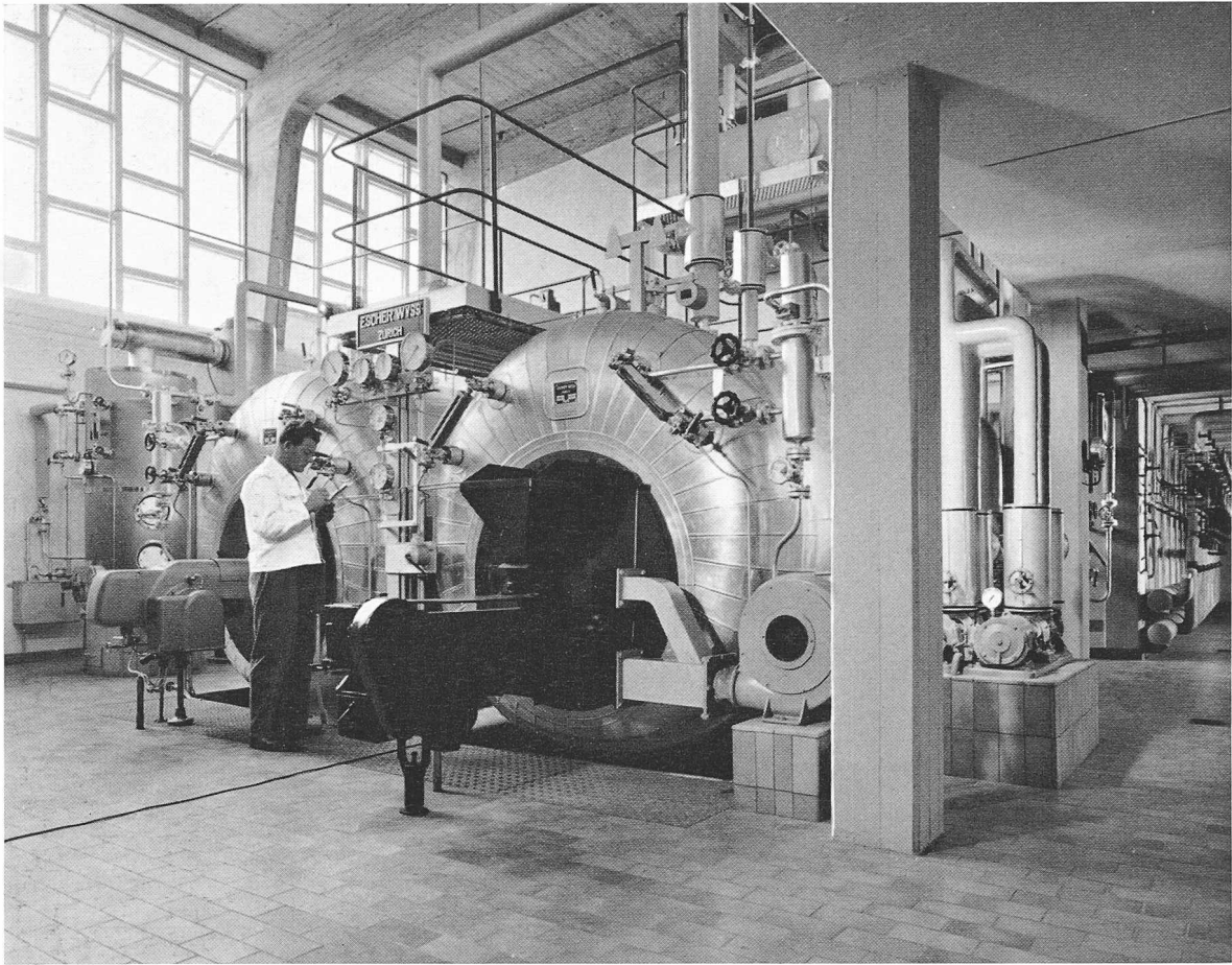
Oben Wärmeeentrale, unten Verteilung für Dampf und Gebäudeheizung
