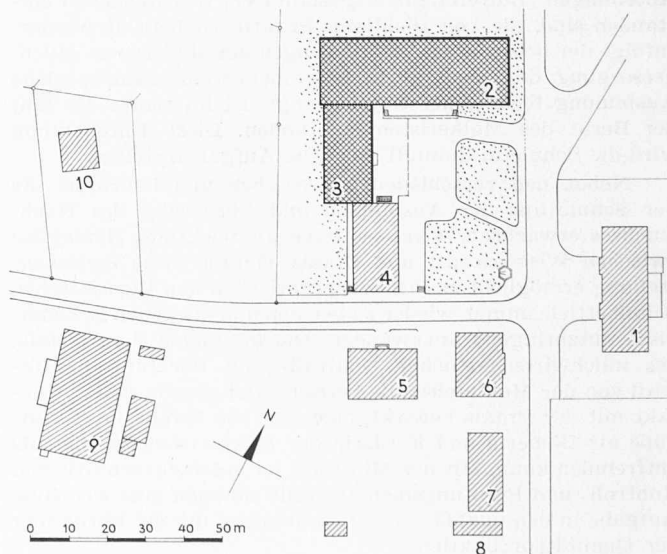
Bild 1. Lageplan der Molkereischule Rütli, Zollikofen, 1:2000. 1 Konviktsgebäude, 2 Neues Betriebsgebäude, 3 Zwischengebäude mit Wärmesentrale und Tiefkühlanlage, 4 Werkstattgebäude, 5 Schulgebäude, 6 Alter Käsespeicher mit Wohnungen, 7 Garagen, 8 Treibhaus und Gemüsegarten, 9 Schweinestallungen, 10 Werkführerwohnhaus
