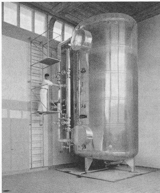
Bild 9. Wärmespeicher für Gebäudeheizung
