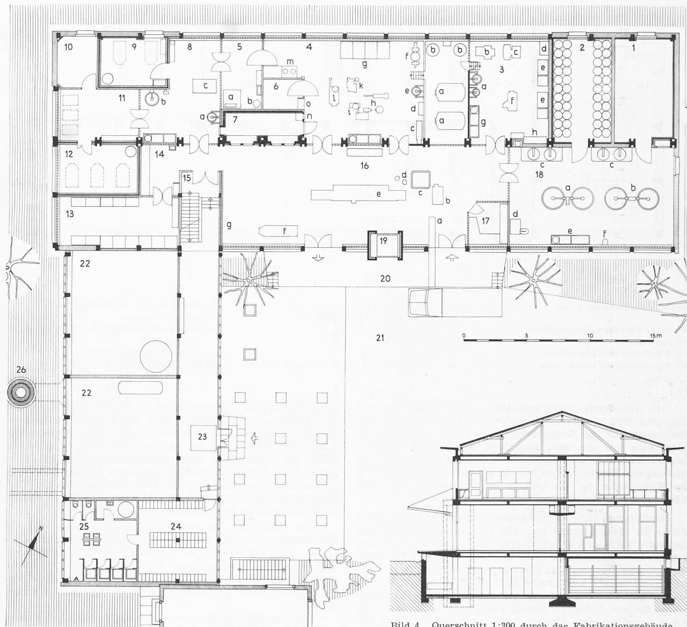
Bild 3. Erdgeschoss 1:300
