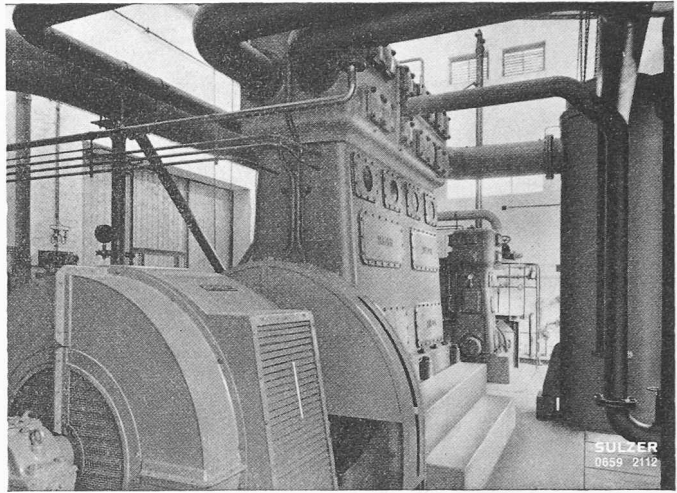
Bild 9. Umlaufkompressor
