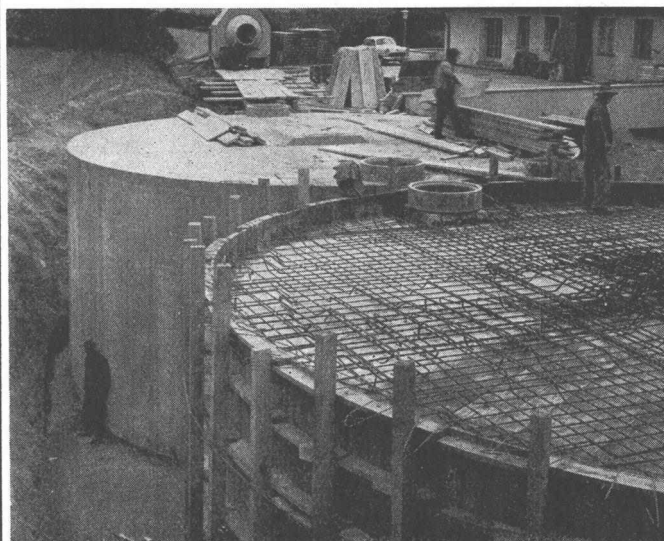
Betonbehälter für Heizöl, Inhalt 500 000 Lt.
