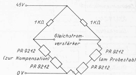
Bild 8. Messbrücke für die zwei auf den Probestab geklebte Dehnungsmessstreifen PR 9212 und deren Kompensation
