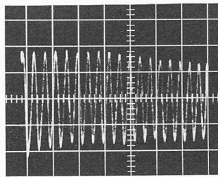
Bild 12. Oszillogramm von J_1(\Delta_1) aus dem Probstab
