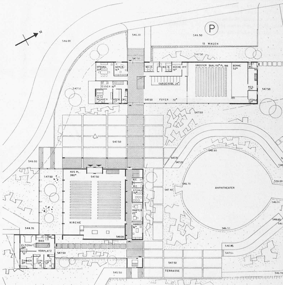
Erdgeschossgrundriss 1:700
