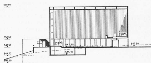
Längsschnitt Kirche
