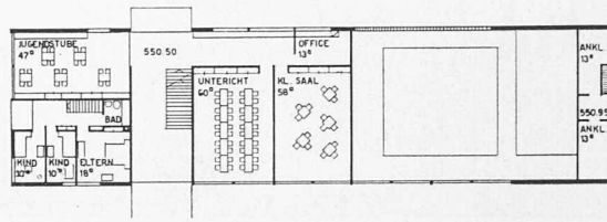
Obergeschoss Kirchgemeindehaus
