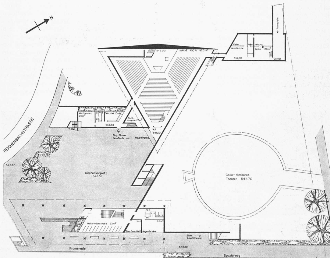
Erdgeschossgrundriss 1:700
