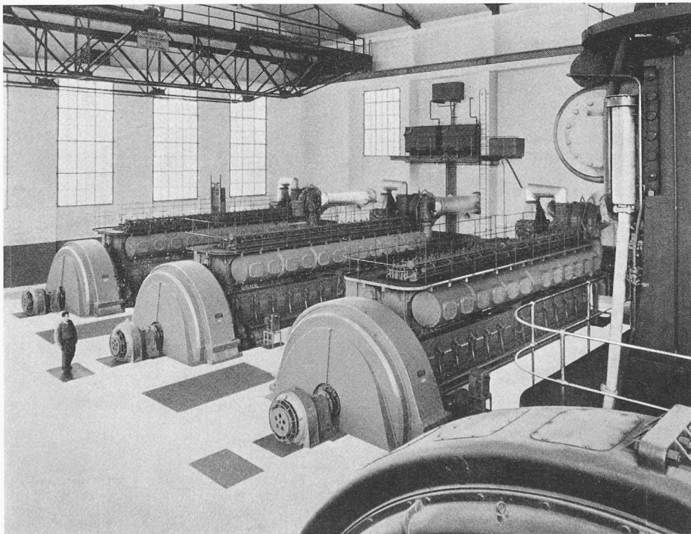
Bild 1. Diesel-elektrische Zentrale «Maigrauge» der Entreprises Fribourgeoises, Fribourg, mit vier Sulzer-Zweitakt-Dieselmotoren von zusammen 26 640 PS
