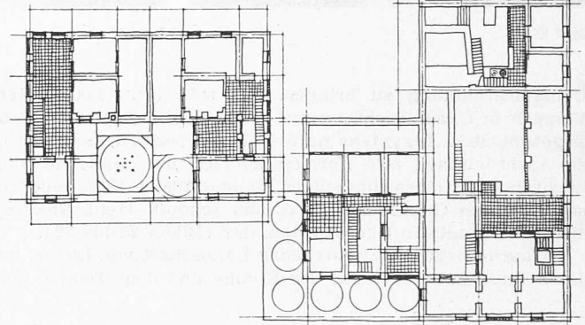
Bild 24 (rechts). Grundriss einer Hauszeile in Gourná Masstab rd. 1:900
