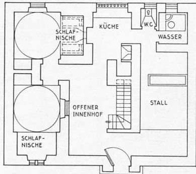
Bild 24 (rechts). Grundriss einer Hauszeile in Gourná Masstab rd. 1:900
