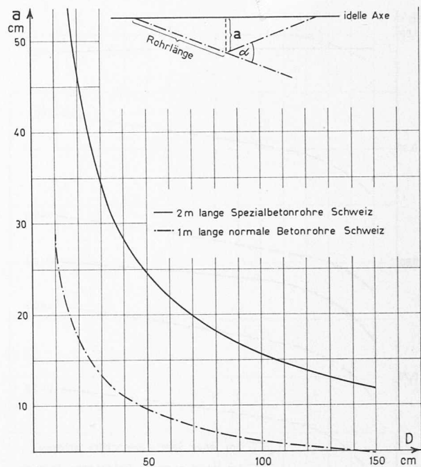
Bild 6. Abweichungen a aus der ideellen Leitungsaxe, berechnet nach Formel \Delta \Delta Z_e = 1 - \cos a (v^2 / 2g)
