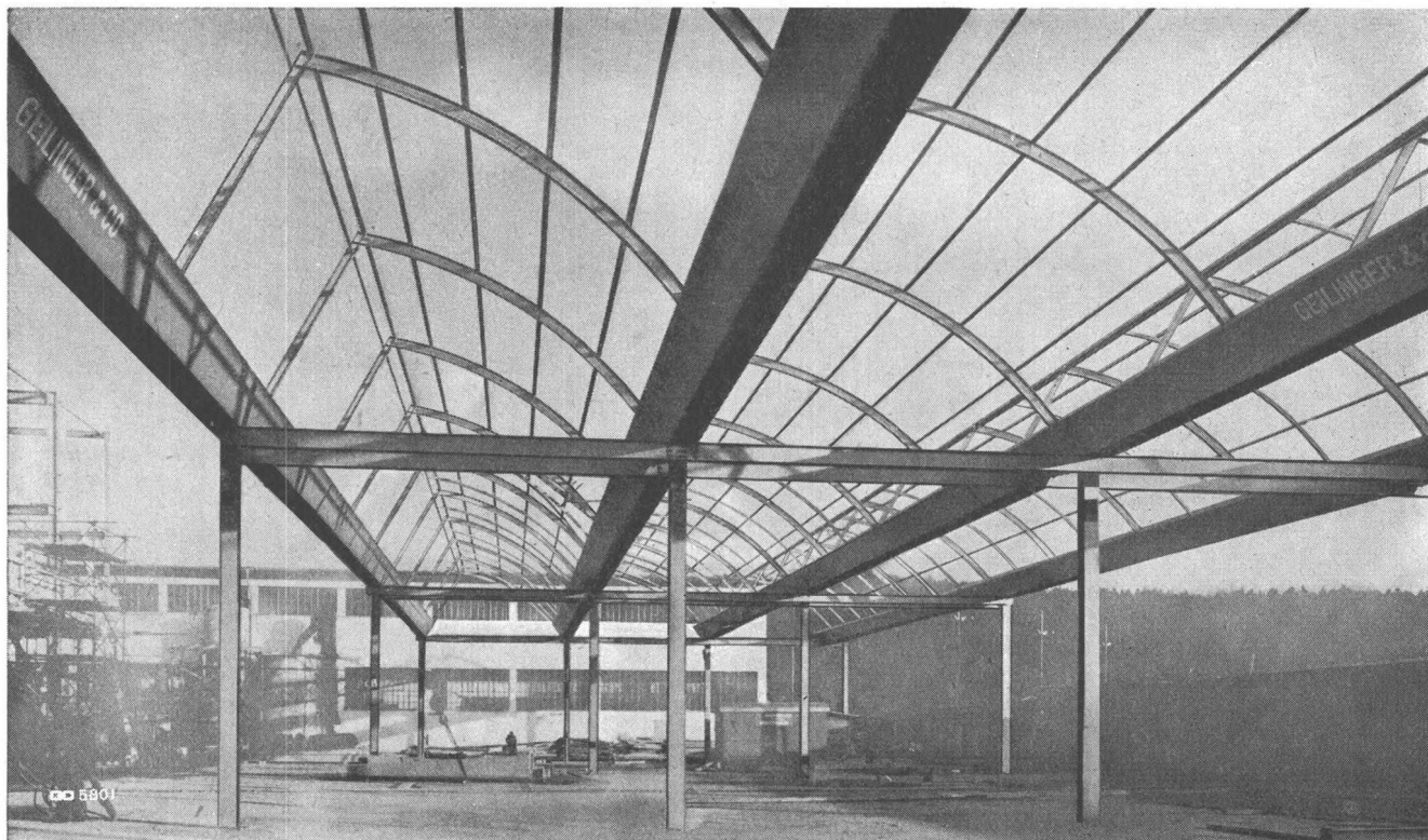
Shedkonstruktion mit rinnenförmigen Hauptträgern (+ Pat. angem.)
