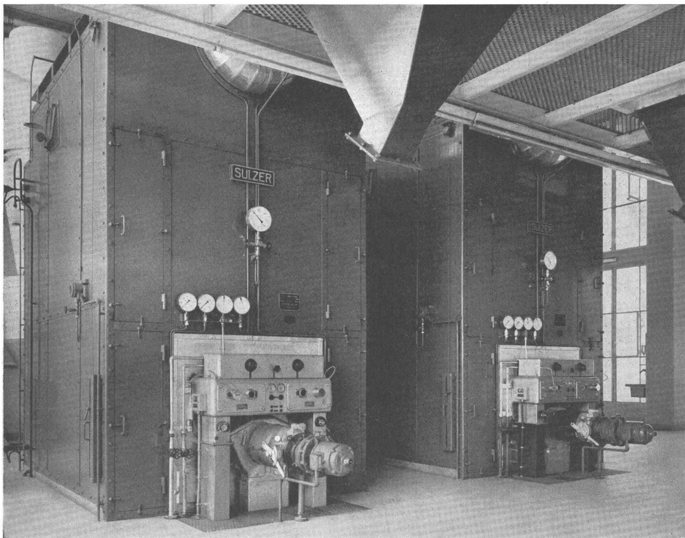
Kleinstrahlungskesselanlage der Firma F. J. Burrus & Cie., Boncourt, mit zwei Einheiten für je 1,25 Mio kcal/h Wärmeleistung, 13 atü Betriebsdruck, eingerichtet für Kohlen- und Ölfeuerung.
