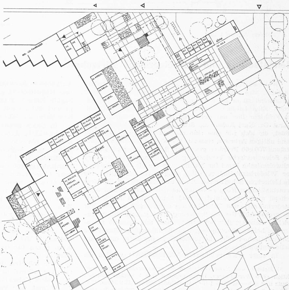
1. Untergeschoss 1:1500
