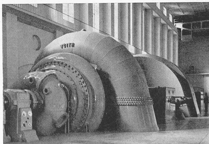
Bild 11. Pumpspeicherwerk Reisch, Maschinenhalle.
