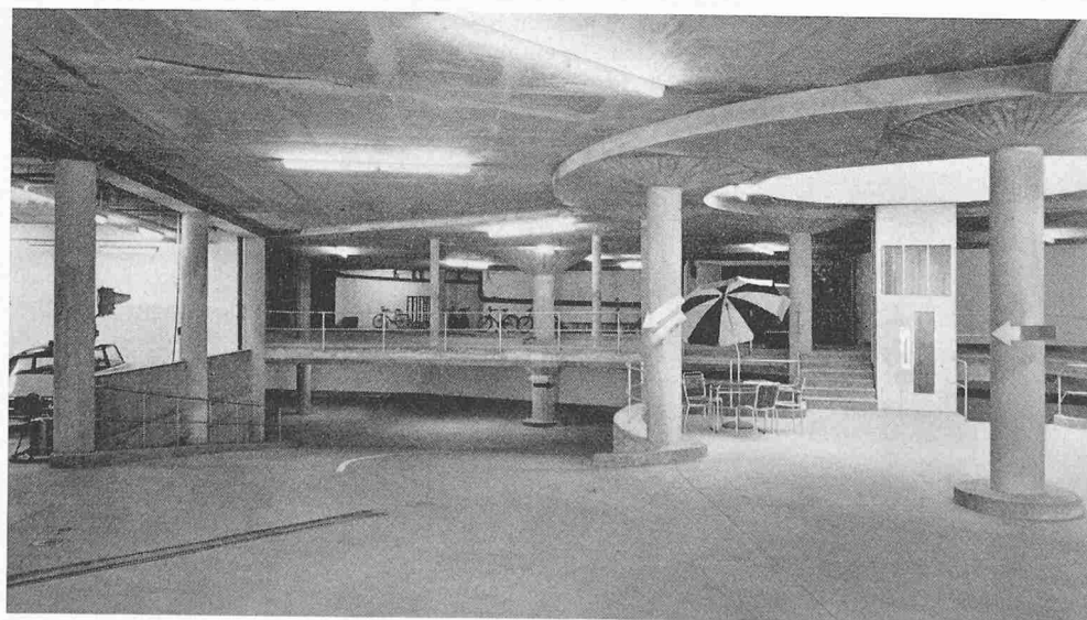
Bild 9. Storch: Einfahrtsrampe mit Ausfahrten auf die um halbe Stockwerkhöhe versetzten Abstellplätze
