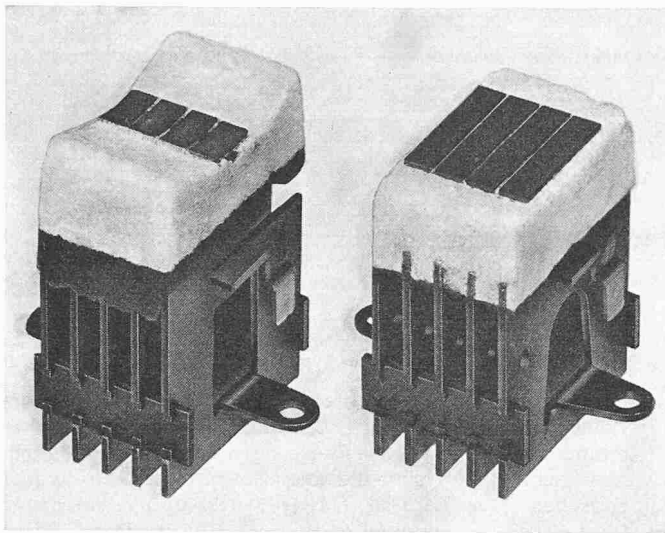
Bild 2. Elektrothermische Kühler (Minnesota Mining and Manufacturing Comp.). An den kalten Lötstellen hat sich Eis angesetzt. Solche Kühler werden z. B. hinter Leuchtstoffröhren eingebaut, um deren Temperatur tief zu halten und damit die Lebensdauer zu vergrössern
