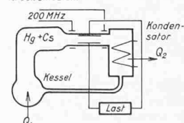
b) Geschlossener Kreislauf mit gasförmigem oder kondensierbarem Arbeitsmedium
