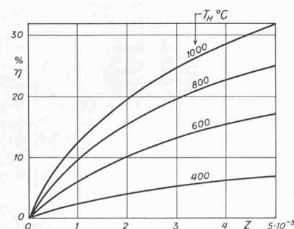
Bild 5 (rechts). Warum eignen sich besonders Halbleiter als Thermolement-Material (nach Justi [4])?
