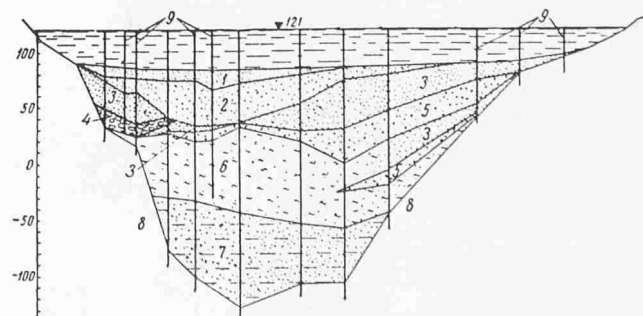
Ueberhöhter Querschnitt durch das Talprofil des Nils an der Dammbaustelle. 1 Feinsand, 2 Mittelsand, 3 Grobsand, 4 Steine, 5 Kies, 6 Grobsand mit Schlammschichten, 7 stark zusammengedrückter Schlamm mit Sandsteinschichten, 8 Granit, 9 Tiefbohrungen
