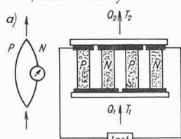
1. Thermoelektrische Generatoren Halbleiter-Thermoelement (Seebeck-Effekt)
