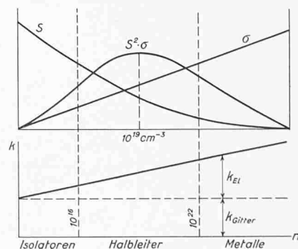
Bild 5 (rechts). Warum eignen sich besonders Halbleiter als Thermolement-Material (nach Justi [4])?
