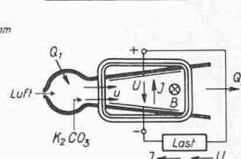
a) Offener Kreislauf
