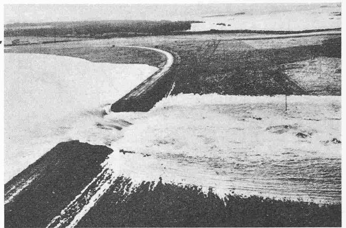
Bild 11. Rincon del Bonete. Gesprengte Bresche im seitlichen Erdstaudamm unter der Zufahrtsstrasse zum Kraftwerk. Dadurch wurde für den See eine geringe zusätzliche Entlastung von rd. 1500 m³/s geschaffen, die jedoch keinen wesentlichen Einfluss hatte (Foto Accion, Montevideo)
