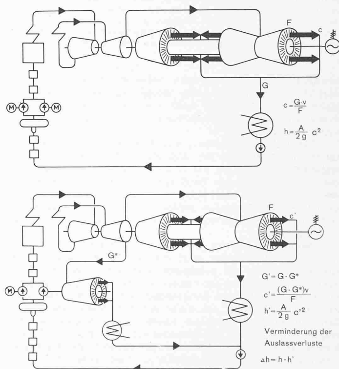
Bild 21. Vergleich zwischen Speisepumpen-Antrieb durch Elektromotor (oberes Bild) mit Antrieb durch Zweigturbine (unteres Bild) wie im Kraftwerk Baudour. Durch die Dampfentnahme aus der Mitteldruck-Turbine für die Zweigturbine wird die durch die Niederdruck-Turbine strömende Dampfmenge vermindert, so dass sich bei Zweigturbinen-Antrieb ein geringerer Auslass-Verlust der letzten Niederdruck-Stufen ergibt (unteres Bild) als bei Elektromotor-Antrieb (oberes Bild). Die Auslassverluste sind durch dicke Pfeile von entsprechender Länge dargestellt
