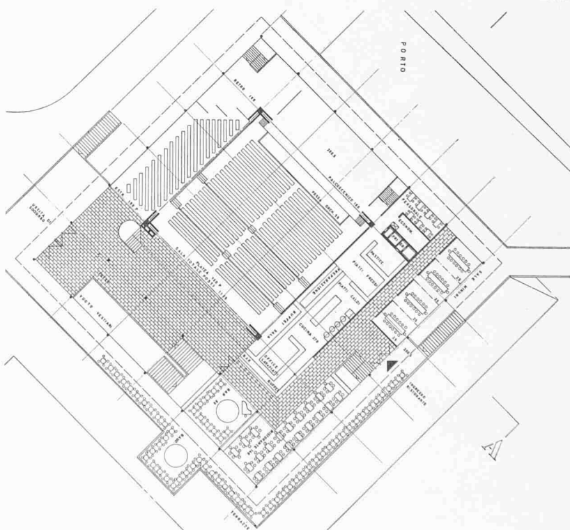
Obergeschossgrundriss, Masstab 1:800
