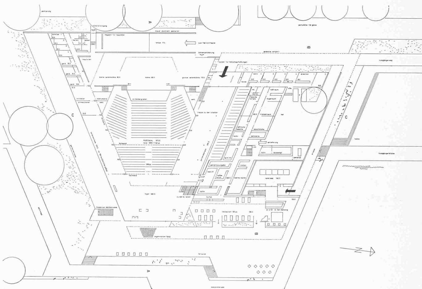
Erdgeschossgrundriss, Masstab 1:800
