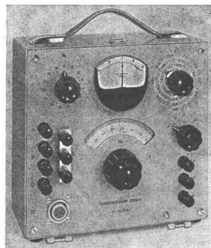
Volltransistor. Präzisions-Messbrücke
