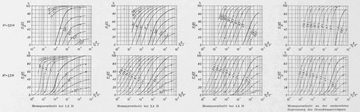
Bild 6. Füllvorgang: Darstellung der Grundwasserpiegellage (Sickerlinie) für beliebige k/(n_s \cdot v) -Werte in den Messquerschnitten (siehe senkrechte Reihen): 1.2 H; 2.4 H; 4.8 H und 8.7 H (= Modellbegrenzung). Die berücksichtigten Grundwassertrögertiefen sind H' = 0.0 H und H' = 1.2 H .
