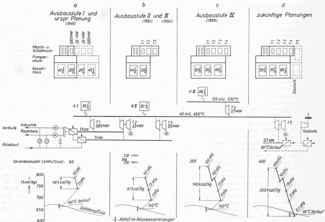
Bild 2. Entwicklungsstufen des Heizkraftwerkes Klagenfurt
