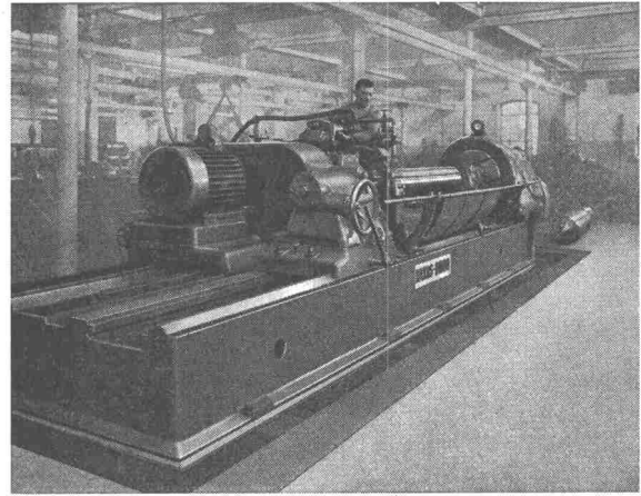
Isolierte Walzenschleifmaschine
