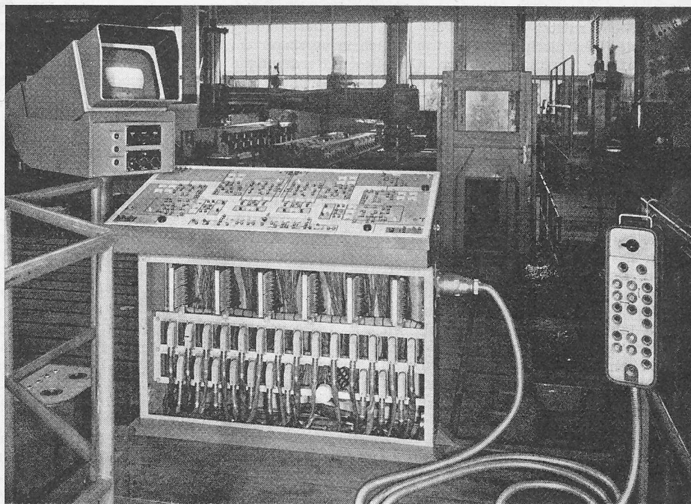
Bild 24. Schalterpult für das Schiess-Hobel- und Fräswerk
