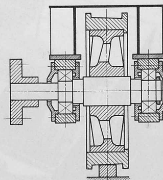
Bild 6. Angetriebene Rolle eines Kranfahrwerks mit Wälzlager. Das Rad ist auf der Achse aufgeschrumpft. Sie ruht in Wälzlager. Antrieb durch die Kupplung. Zweiteilige Rolle mit konischer Lauffläche
