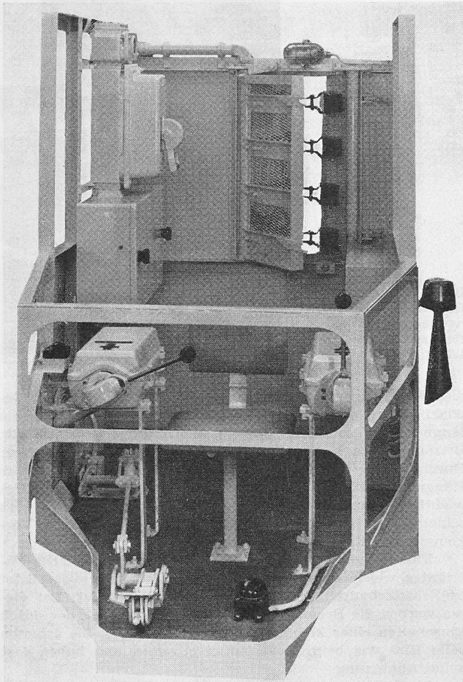
Bild 10. Kabine eines alten Giessereikrans mit Kontrollsteuerung
