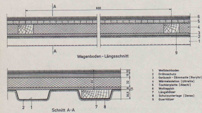
Bild 6. Schnitte des Fußbodens im Abteil Maßstab 1:5
