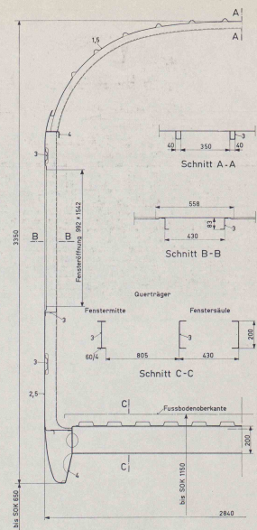
Bild 3. Kastenquerschnitt eines Personenwagens. Die eingetragenen Zahlen geben die Blechdicken in mm an, Maastab 1:20
