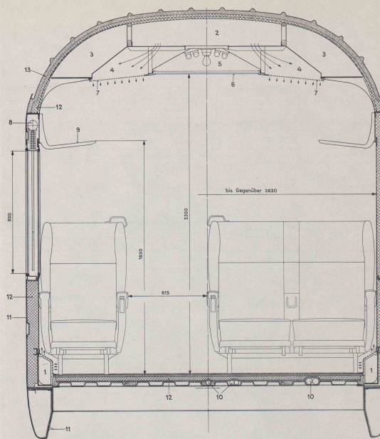
Bild 7. Querschnitt des Wagenkastens mit Isolation und Luftkanälen. Masstab 1:17
