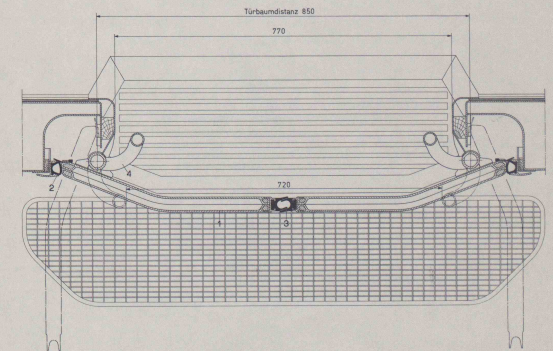
Bild 10 (unten). Horizontalschnitt 1:7 durch die Einstiegtüre 1 Türflügel 2 Gummischlauchdichtung 3 Gummidichtprofil 4 Handgriff
