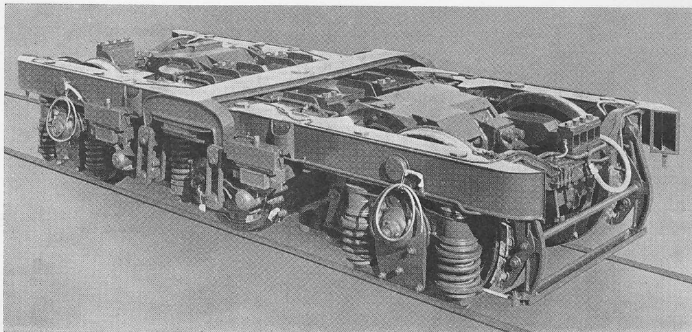
Bild 25 (rechts). Ansicht des dreiachsigen Triebgestells, Radstand 3,80 m
