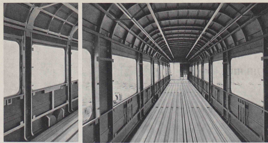
Bild 3. Innenansicht zur Seitenwand Unter dem Fenster sieht man die Eintrittsstutzen zu den Luftkanälen an der Seitenwand
