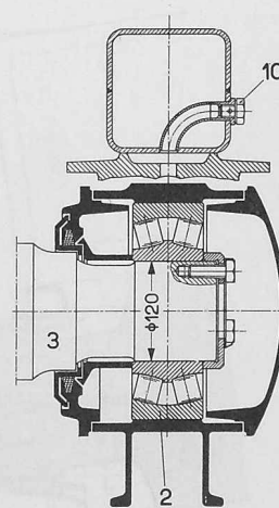
Schnitt A-B
