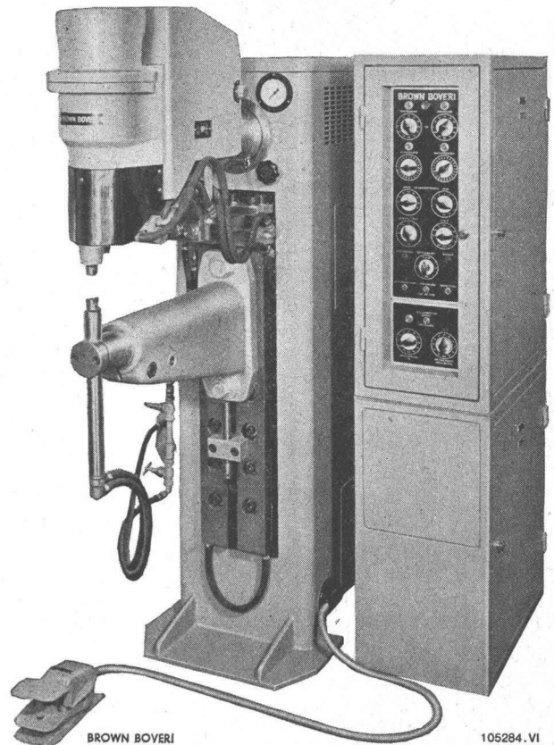
Universelle druckluftbetätigte und röhrengesteuerte Punktschweisssmaschine. Sie eignet sich gleichermassen für das Einzelpunktschweissen hoher Qualität und auch zum Steppen und für kleinere Buckelschweisssarbeiten. Die zugeordnete elektronische Steuerung erlaubt nicht nur die Funktionen Vorpresen, Schweissen, Nachpressen und Repetieren, sondern auch das Mehrimpulsschweissen. Zudem kann mit Schwellstrom, auch Modulation oder «slope control» genannt, geschweisst werden und der Schweissstrom durch Zündpunktverschiebung an den Ignitrons geregelt werden.
