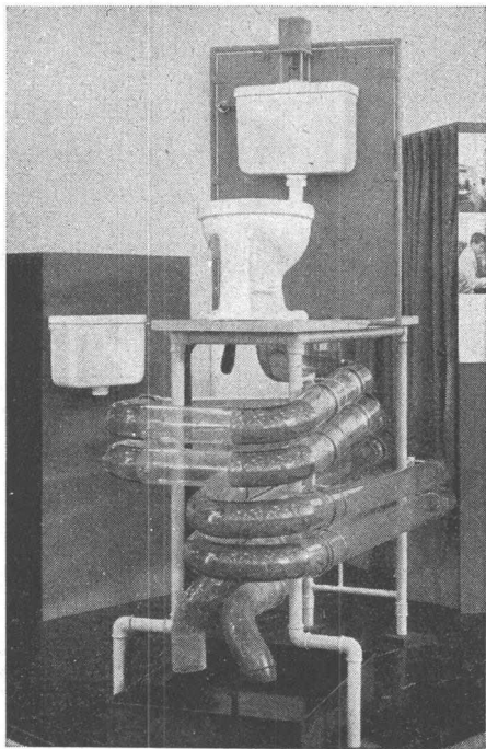
Ansicht der Versuchsanlage mit insgesamt 20 m glasklaren Rohren zur Demonstration der Ueberlegenheit von Spülkasten-Spülung gegenüber Spülhahn-Spülung
