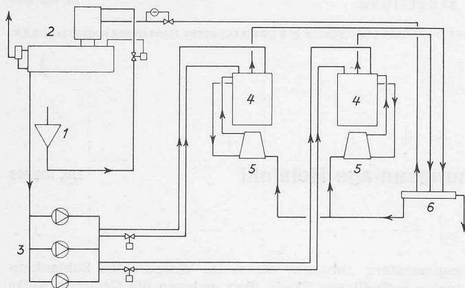
Bild 2. Thermisches Schema
