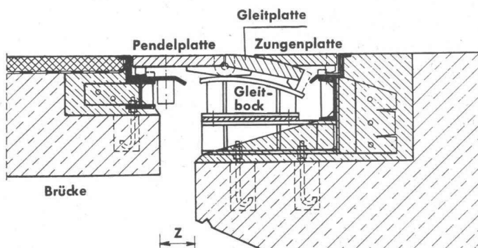
Querschnitt durch einen Fahrbahnübergang (normale Ausführung)
