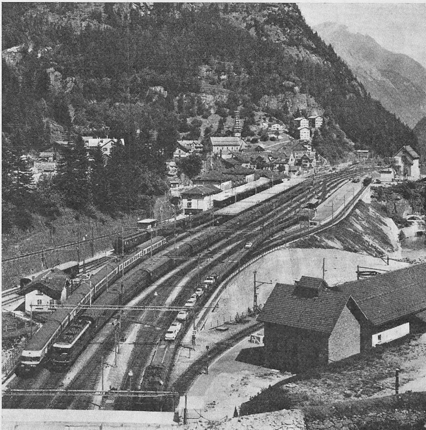
Bild 3. Die neue Gleisanlage in Göschenen nach Inbetriebnahme des Blocks im Tunnel
