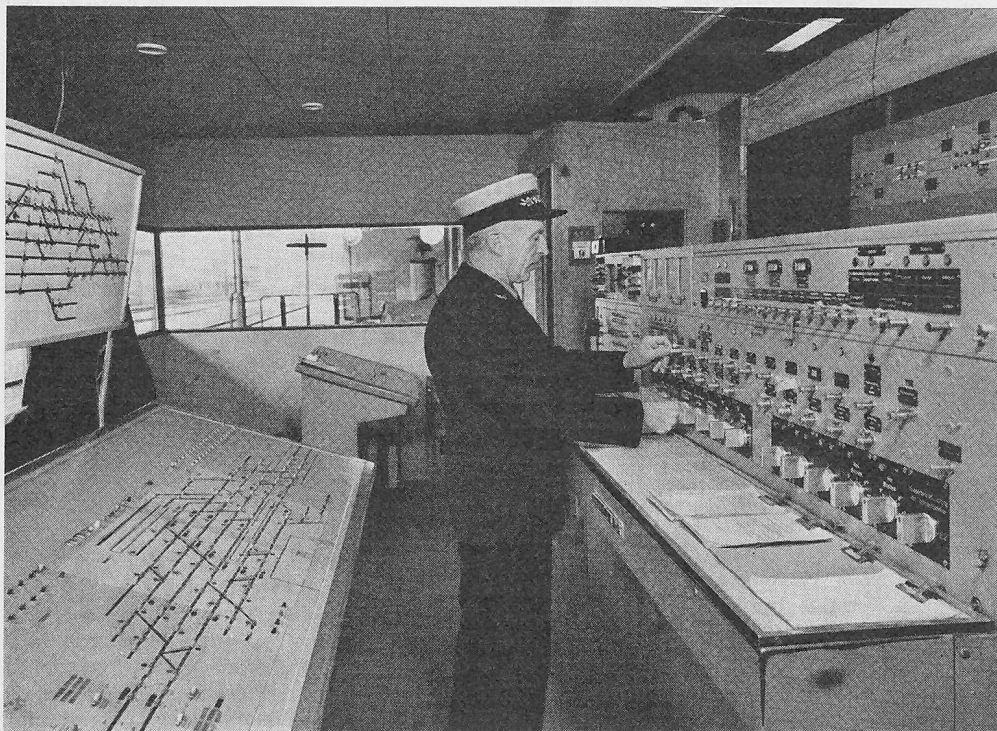
Bild 2. Stellwerkraum während des Umbaus. Links im Vordergrund: Neues Domino-Bedienungspult, links oben: Provisorische Gleistafel für die Durchprüfung der neuen Anlage, im Hintergrund links: Provisorisches Bedienungspult für die Umbauweichen im Tunnel, rechts vorn: Altes Schalterwerk Bauart Integra, darüber alte Gleistafel für Meldungen von der Tunnelstation Gotthard
