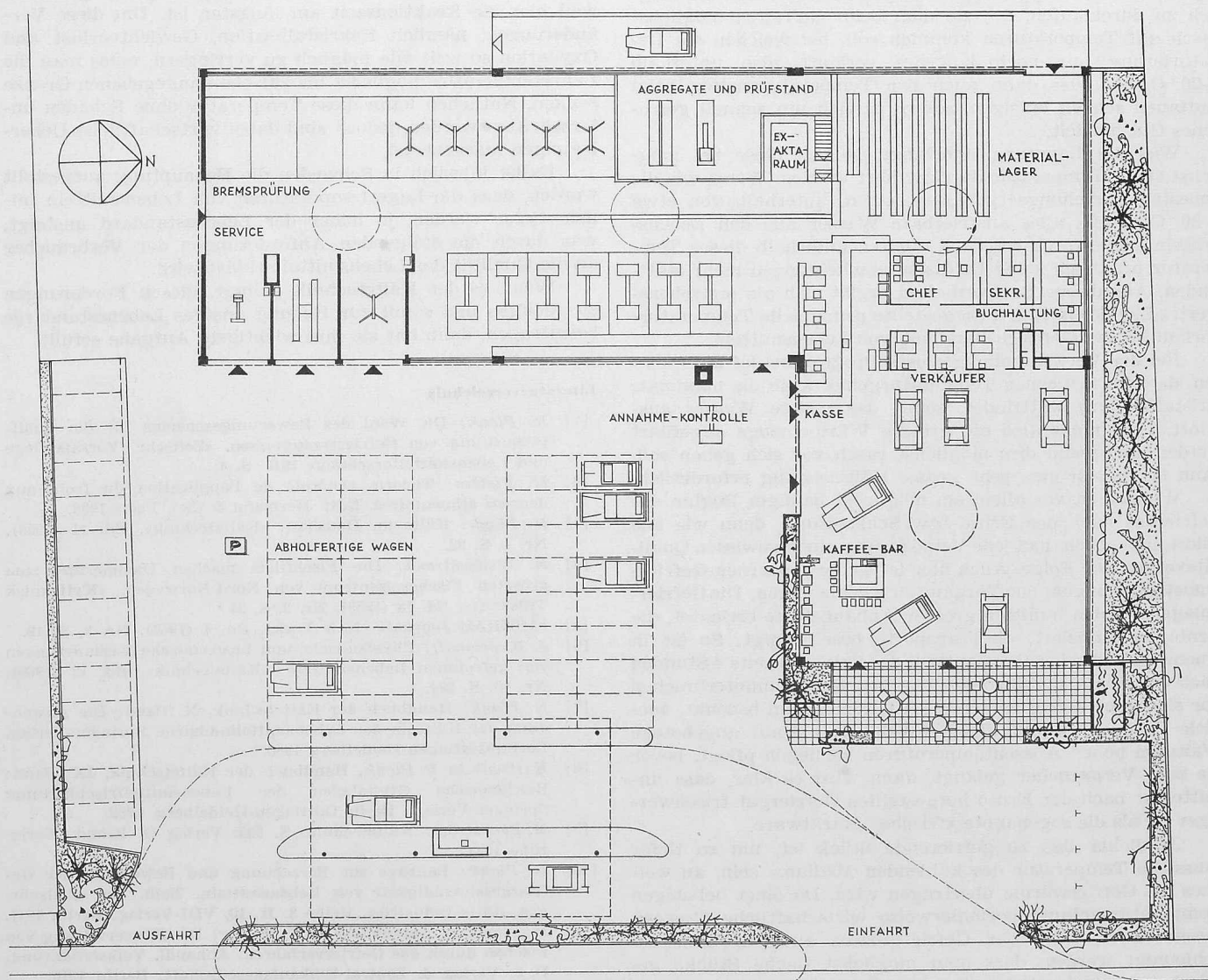
Erdgeschoss, Masstab 1:500
