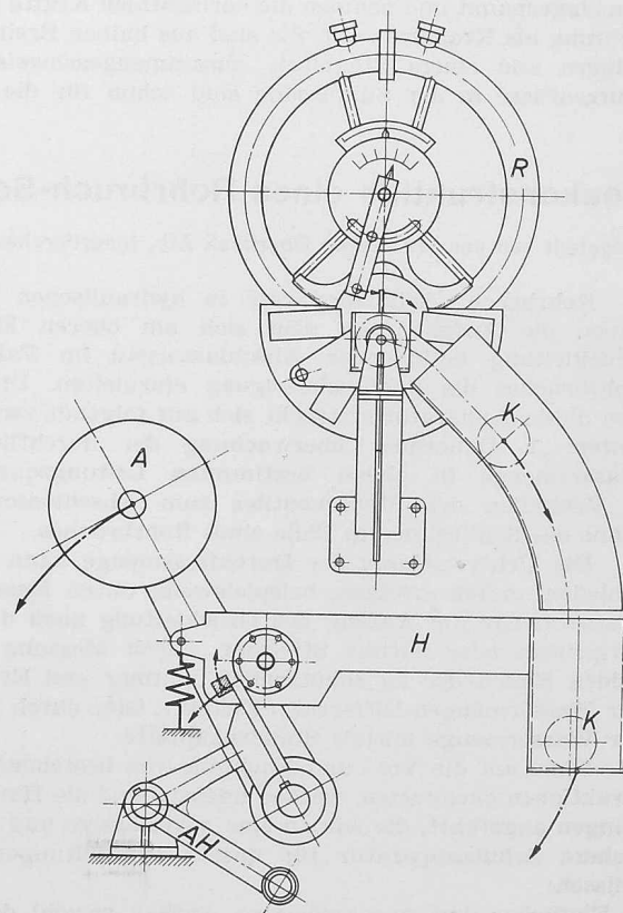
Bild 4. Auslösemechanismus mit Abrollkugel K, Auslösehebel H, Auslösegewicht A und Arretierung AH
