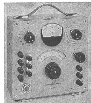
Volltransistor. Präzisions-Messbrücke
