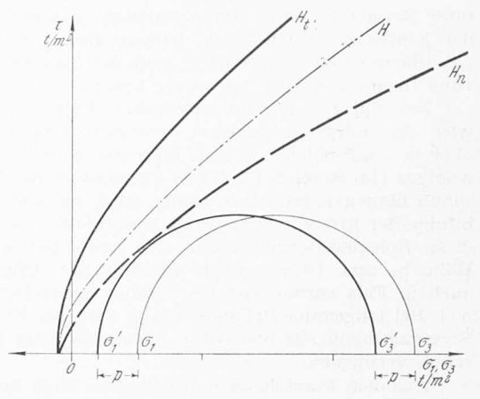
Bild 12. Mohrscher Kreis bei überlagertem Kluftwasserdruck
