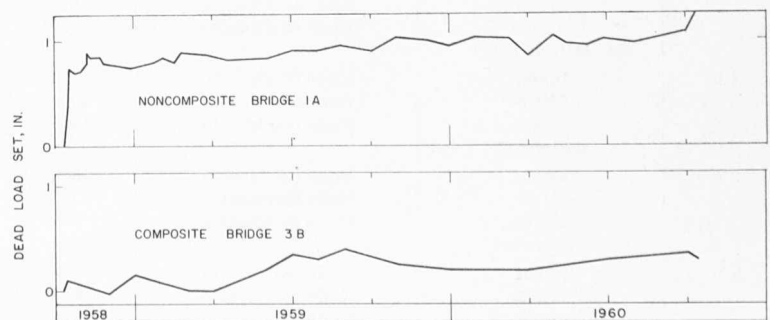
Bild 9. Durchbiegung in Funktion der Zeit für den mittleren Hauptträger der Stahlbrücken. Dead load set = Durchbiegung infolge Eigengewicht (1 in = 2,54 cm); Noncomposite = ohne Verbund; Composite = mit Verbund
