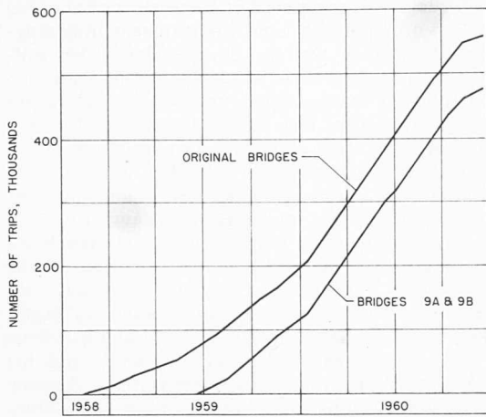
Bild 6. Totale Anzahl Durchgänge der normalen Versuchsfahrzeuge
