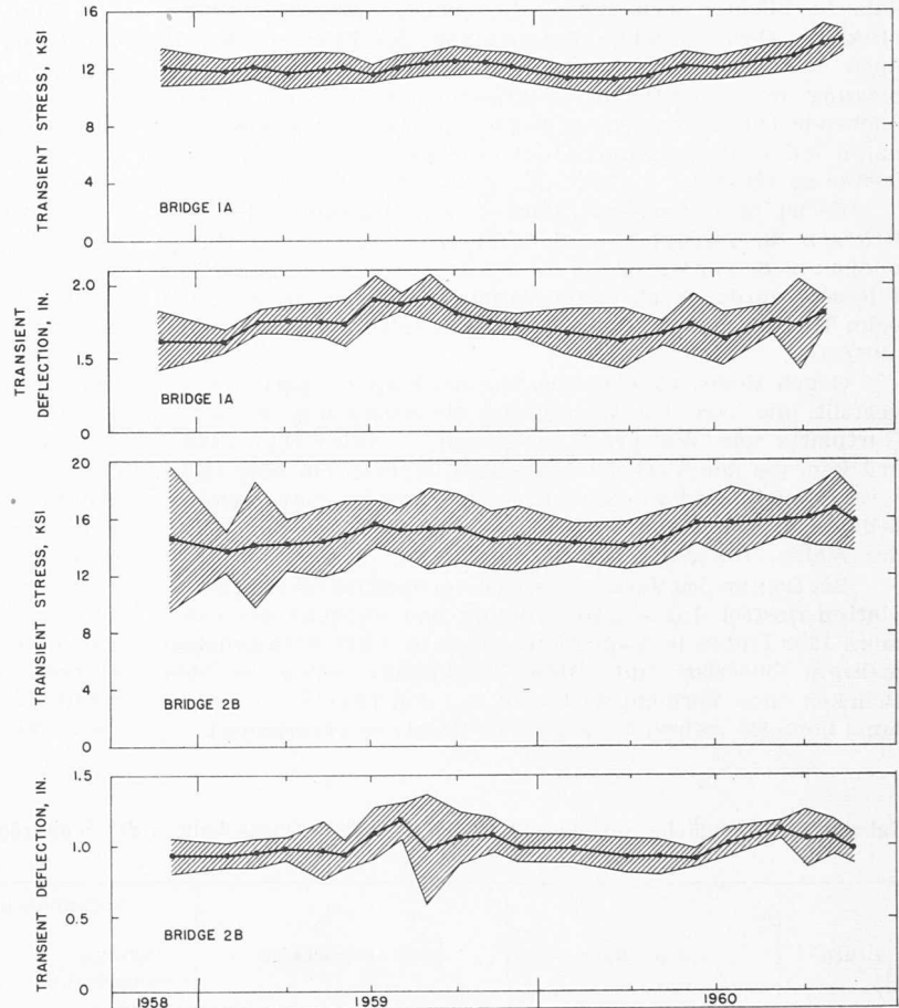
Bild 7 (rechts). Spannung und Durchbiegung in Funktion der Zeit für den mittleren Hauptträger der Stahlbrücken 1 A und 2 B. Transient deflection = kurzfristige Durchbiegung (1 in = 2,54 cm); Transient stress = kurzfristige Spannung (1 ksi = 70,3 kg/cm 2 )
