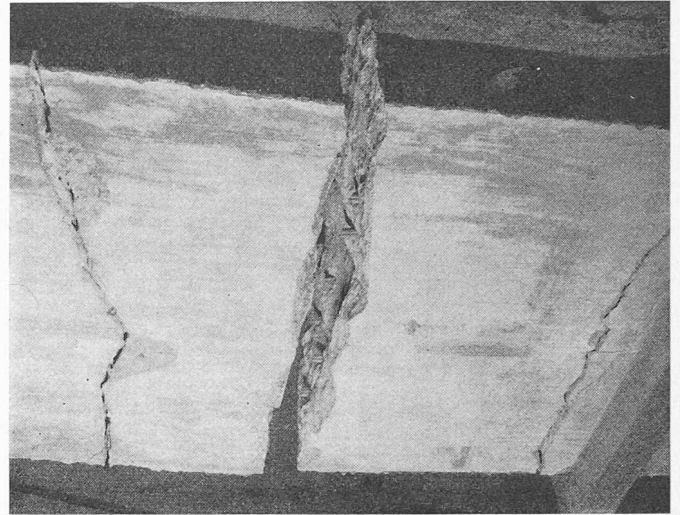
Bild 19. Gebrochene Litzen in der Spannbetonbrücke 6 A
