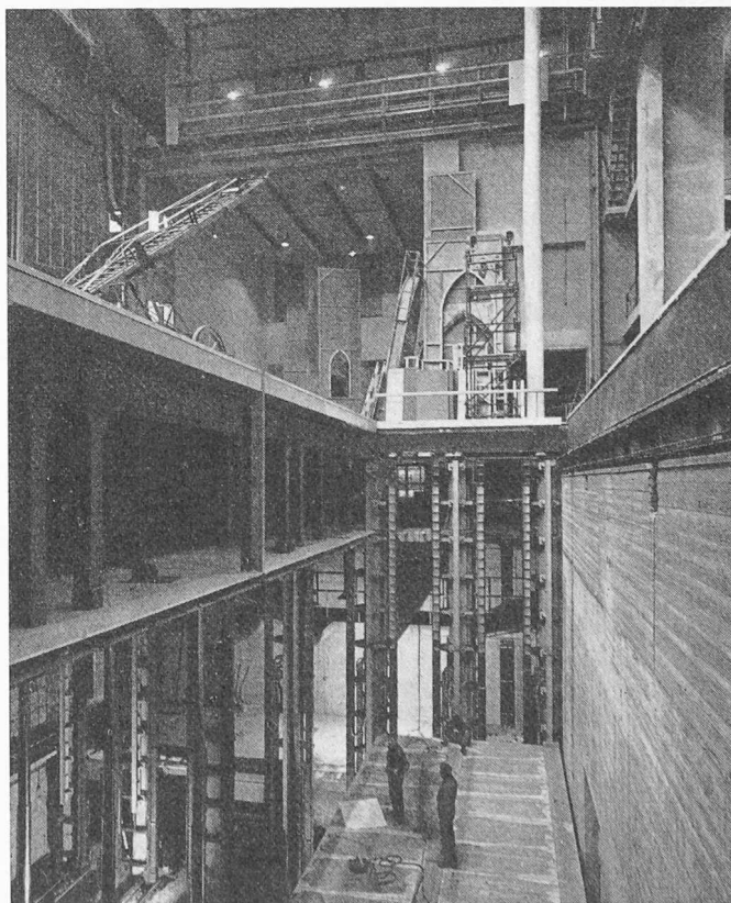
Mechanische Bühneneinrichtung. Blick auf die Hebebühnen und in eine Seitenbühne (im Hintergrund des oberen Bildteils)
