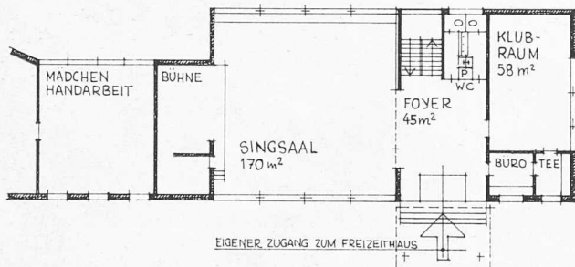
Erdgeschoss 1:400
