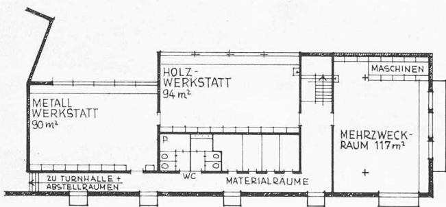
Untergeschoss 1:400
