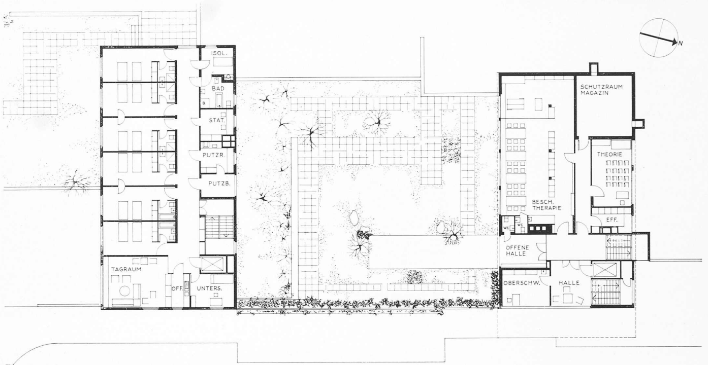
Erstes Obergeschoss 1 : 400
