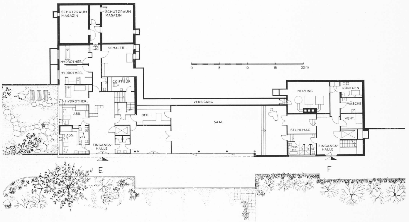
Erdgeschoss 1 : 400
