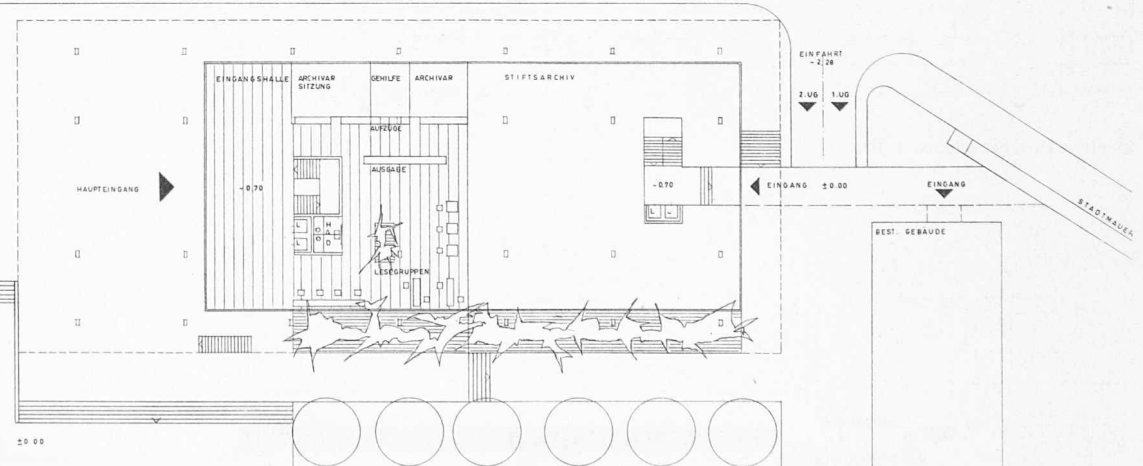
Grundrisse 1:700
