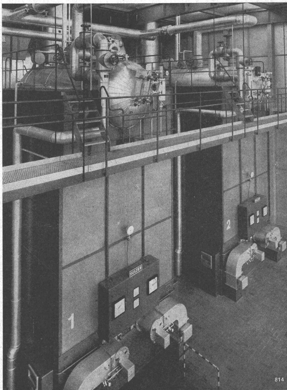
Zwei Strahlungskessel Typ C, Leistung je 6,4 Millionen kcal/h, Betriebsdruck 13 atü, mit Hauptdampf- und Speiseleitungen. Beide Kessel sind mit einer Ölfeuerung ausgerüstet und der Kessel links zusätzlich noch mit einer Abfallverbrennung.
